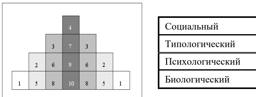
Рис. 9. Четырехуровневый субъект
