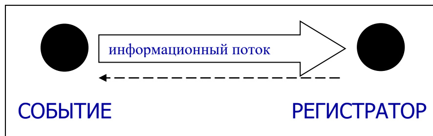
Рис. 3. Информационный процесс
