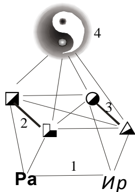
Рис. 4. Базис Юнга-Аугустиновичюте:
