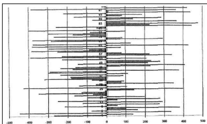
Рис. 3. Среднее значение x в контрольных измерениях.
